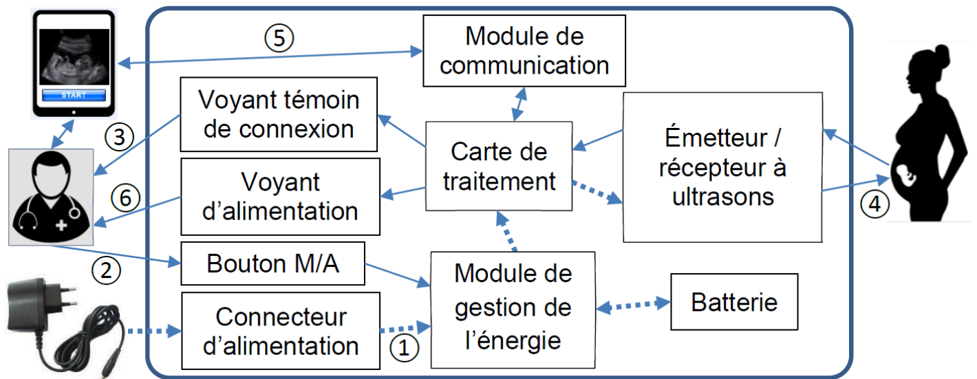
Document 1 : principe de fonctionnement d'un échographe portable.
